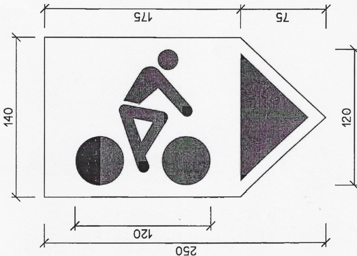
CYKLOSMEROVKA, M1:2
