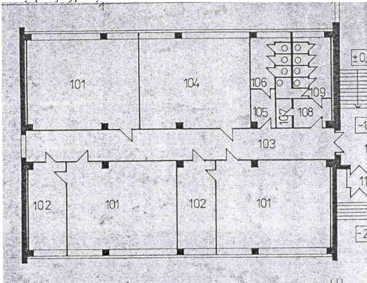
Príloha 3.2. Pôdorys prenajatej plochy
