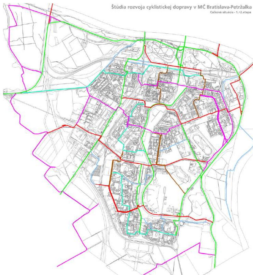
Obr. 2 – 1.+2. etapa návrhu cyklistických trás
